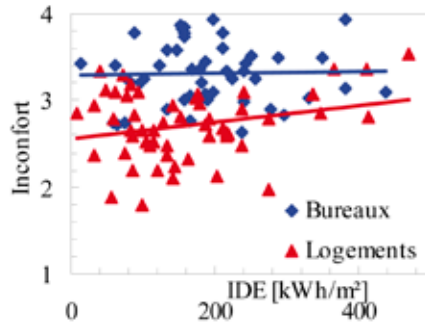
Figure 1: Chaque bâtiment évalué est représenté par un point dont son indice de dépense d'énergie en abscisse et l'inconfort global évalué par les occupants sur une échelle allant de 1 (confortable) à 7 (totalement inconfortable).
