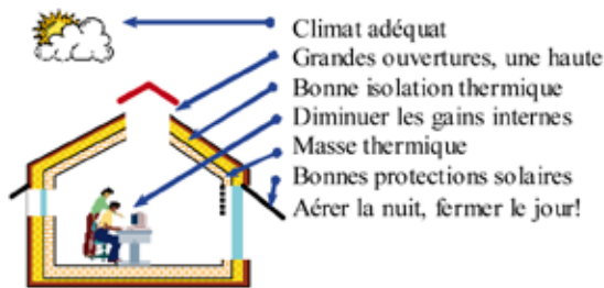
Figure 7: Conditions nécessaires pour un refroidissement passif efficace
