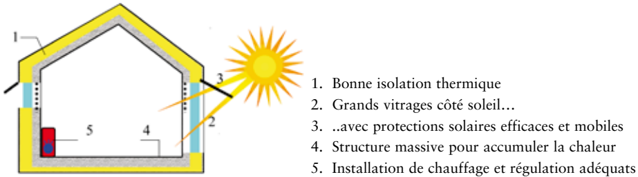
Figure 4: Principes du chauffage solaire passif
